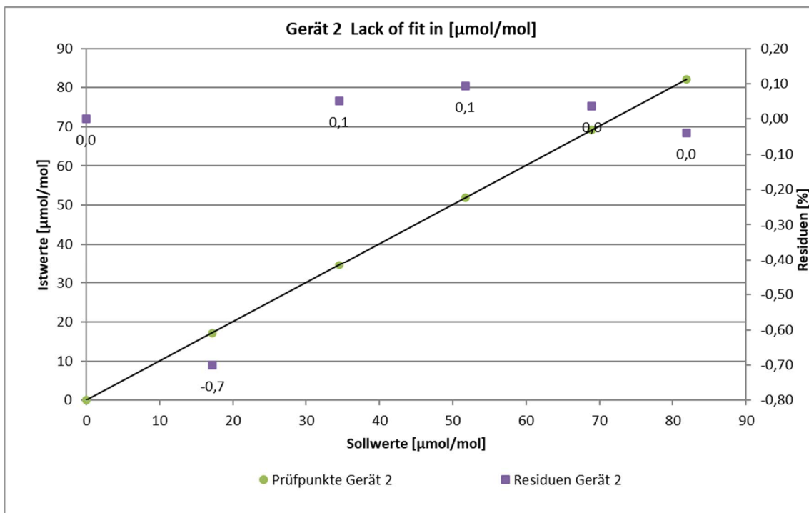
Abbildung 10: Analysenfunktion aus den Gruppenmittelwerten für Gerät 2
