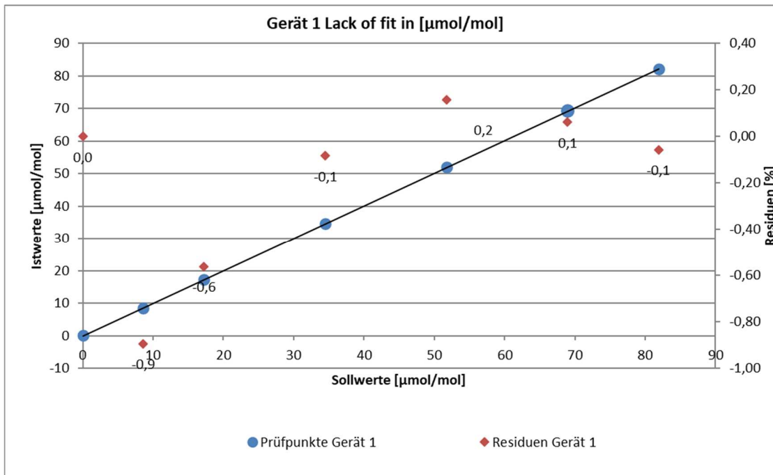
Abbildung 13: Analysenfunktion aus den Gruppenmittelwerten für Gerät 1 (EN 14626:2024)
