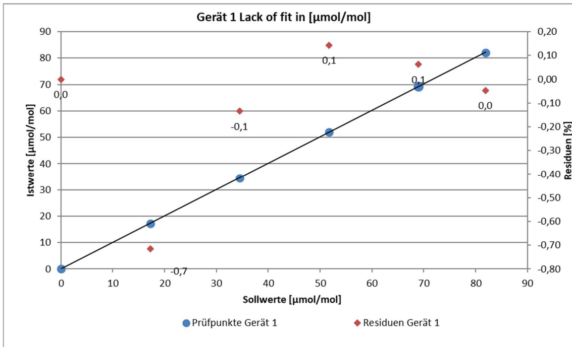
Abbildung 9: Analysenfunktion aus den Gruppenmittelwerten für Gerät 1
