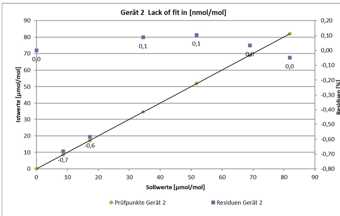
Abbildung 14: Analysenfunktion aus den Gruppenmittelwerten für Gerät 2 (EN 14626:2024)
