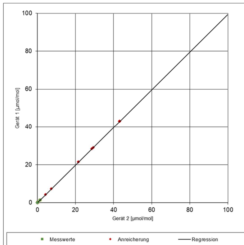
Abbildung 15: Grafische Darstellung der Vergleichsstandardabweichung für CO im Feld
