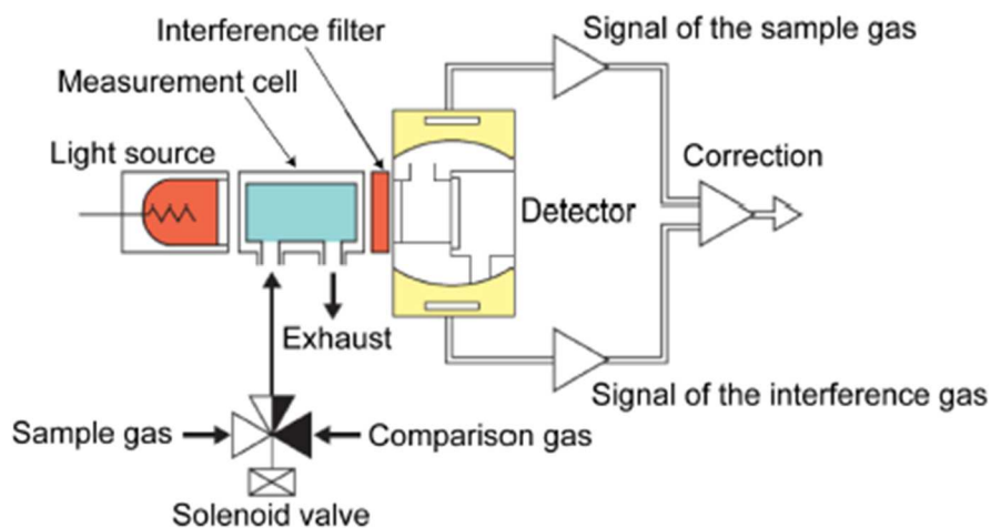
Abbildung 2: NDIR Messverfahren
