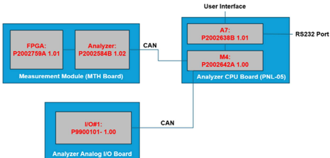
Abbildung 3: Softwareübersicht
