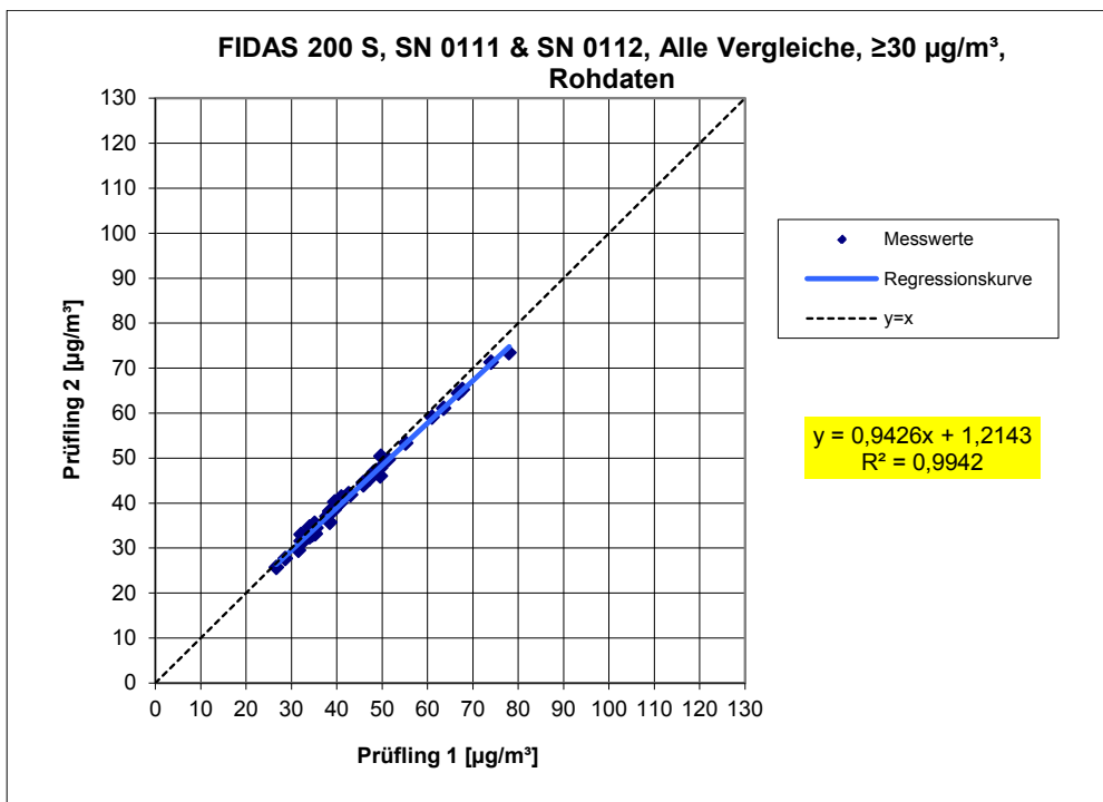
Abbildung 110: Ergebnis der Parallelmessungen mit den Testgeräten SN 0111 / SN 0112, Messkomponente PM 10 , alle Standorte (D+UK), Werte ≥ 30 µg/m³, PM_ENVIRO_0011
