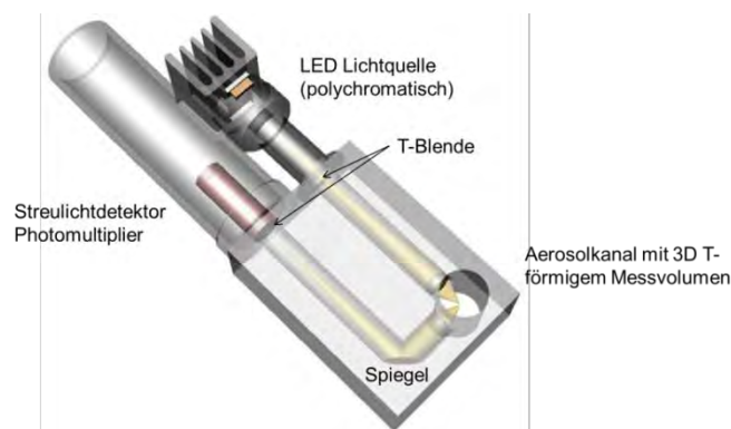
Abbildung 1: Aufbau des Sensors des Fidas® Messsystems
