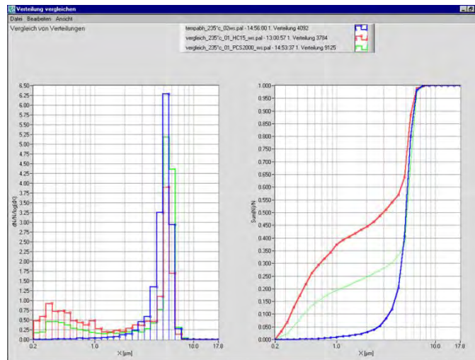
Abbildung 5: Vergleich eines optischen Streulichtspektrometers mit einfacher Rechteckblende (HC15, rot) mit einem opt. Streulichtspektrometer mit T-Blende (welas®, blau) unter Aufgabe von monodispersen 5 µm Partikeln
