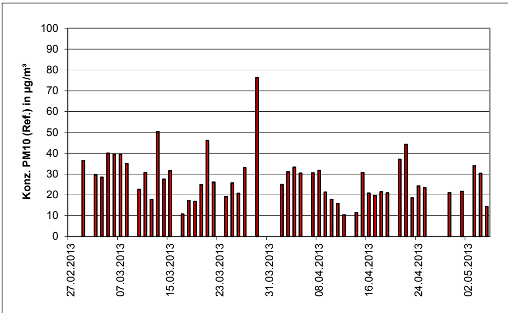
Abbildung 31: Verlauf der PM 10 -Konzentrationen (Referenz) am Standort „Bonn, Winter“
