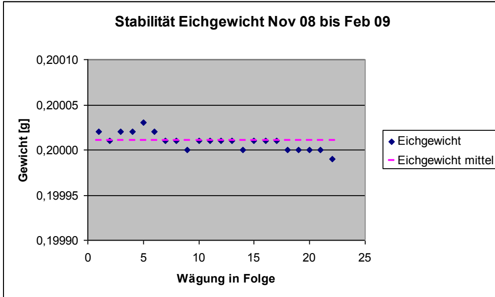
Abbildung 102: Stabilität Eichgewicht
