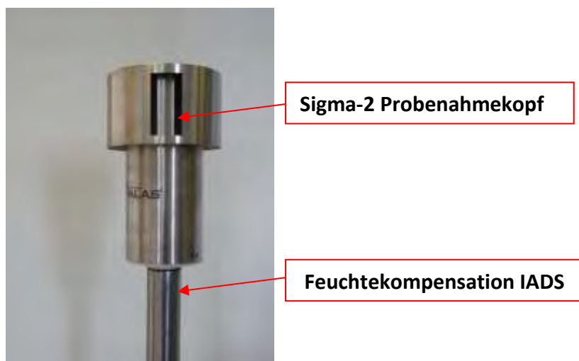
Abbildung 44: Sigma-2 Probenahmekopf
