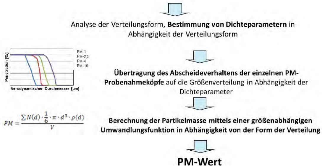
Abbildung 8: Überblick über die einzelnen Messschritte Fidas® 200 S bzw. Fidas® 200
