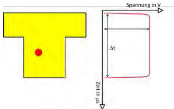
Abbildung 42: Messung des Streulichtsignals am Einzelpartikel. Gemessen wird die Amplitude und die Signallänge
