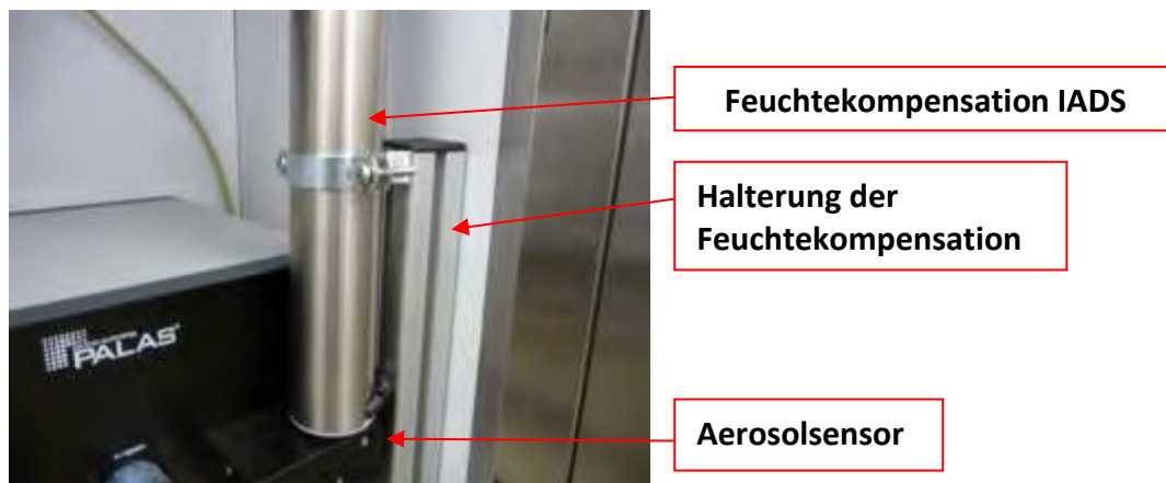
Abbildung 45: Fidas® Steuereinheit, Aerosolsensor mit IADS
