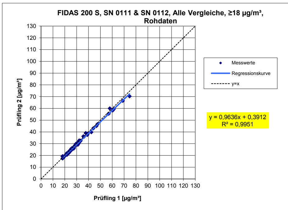
Abbildung 52: Ergebnis der Parallelmessungen mit den Testgeräten SN 0111 / SN 0112, Messkomponente PM 2,5 , alle Standorte, Werte \geq 18 \mu\text{g}/\text{m}^3 , PM_ENVIRO_0011
