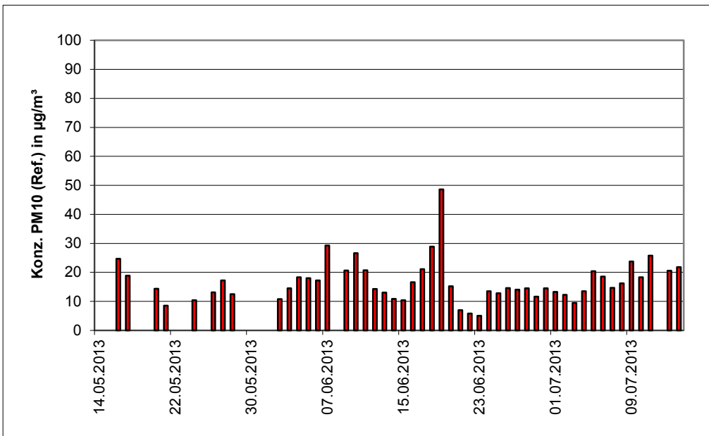
Abbildung 32: Verlauf der PM 10 -Konzentrationen (Referenz) am Standort „Bornheim, Sommer“
