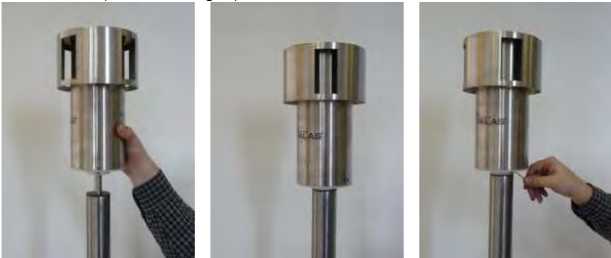
Abbildung 22 A-C: Anbringen des Sigma-2 Probenahmekopfes
