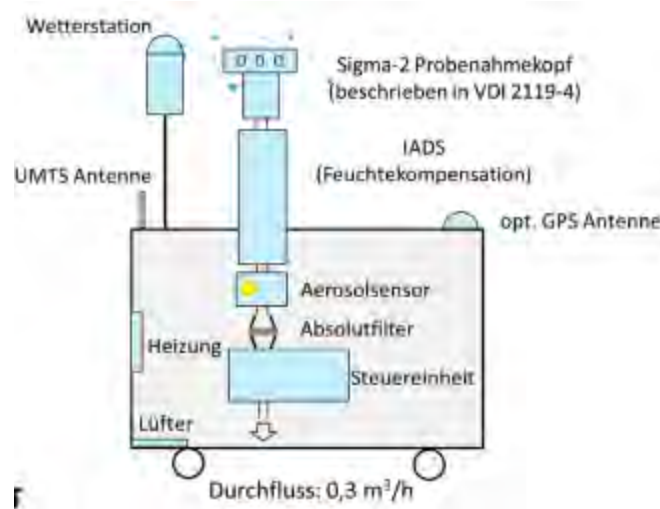
Abbildung 7: Schematischer Aufbau Fidas® 200 S
