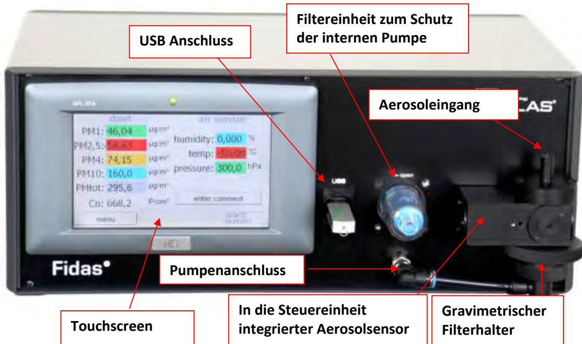
Abbildung 2: Vorderseite der Fidas® Steuereinheit
