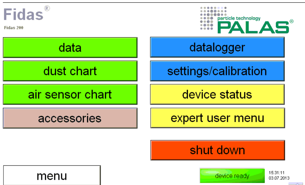
Abbildung 18: Hauptmenü
