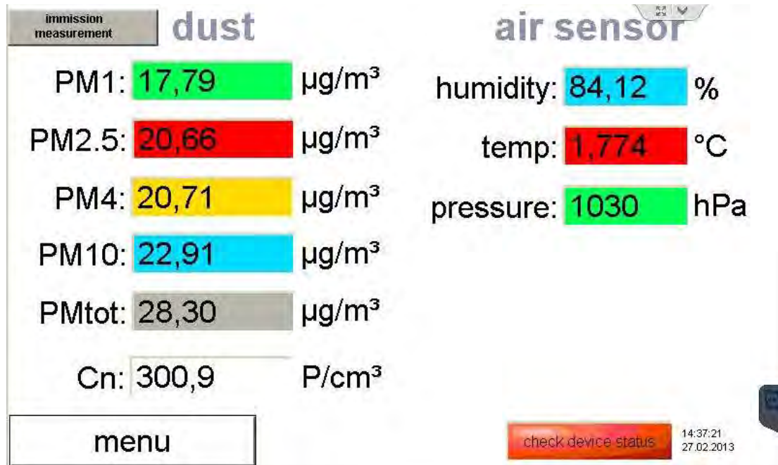
Abbildung 3: „data“ - Datenübersicht
