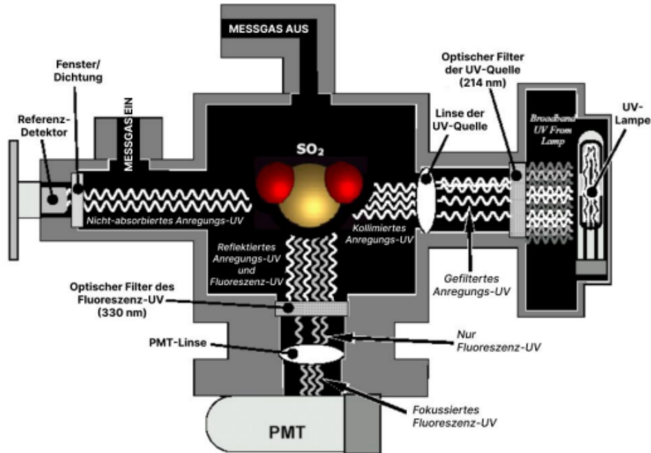
Abbildung 2: N100 UV Lichtpfad
