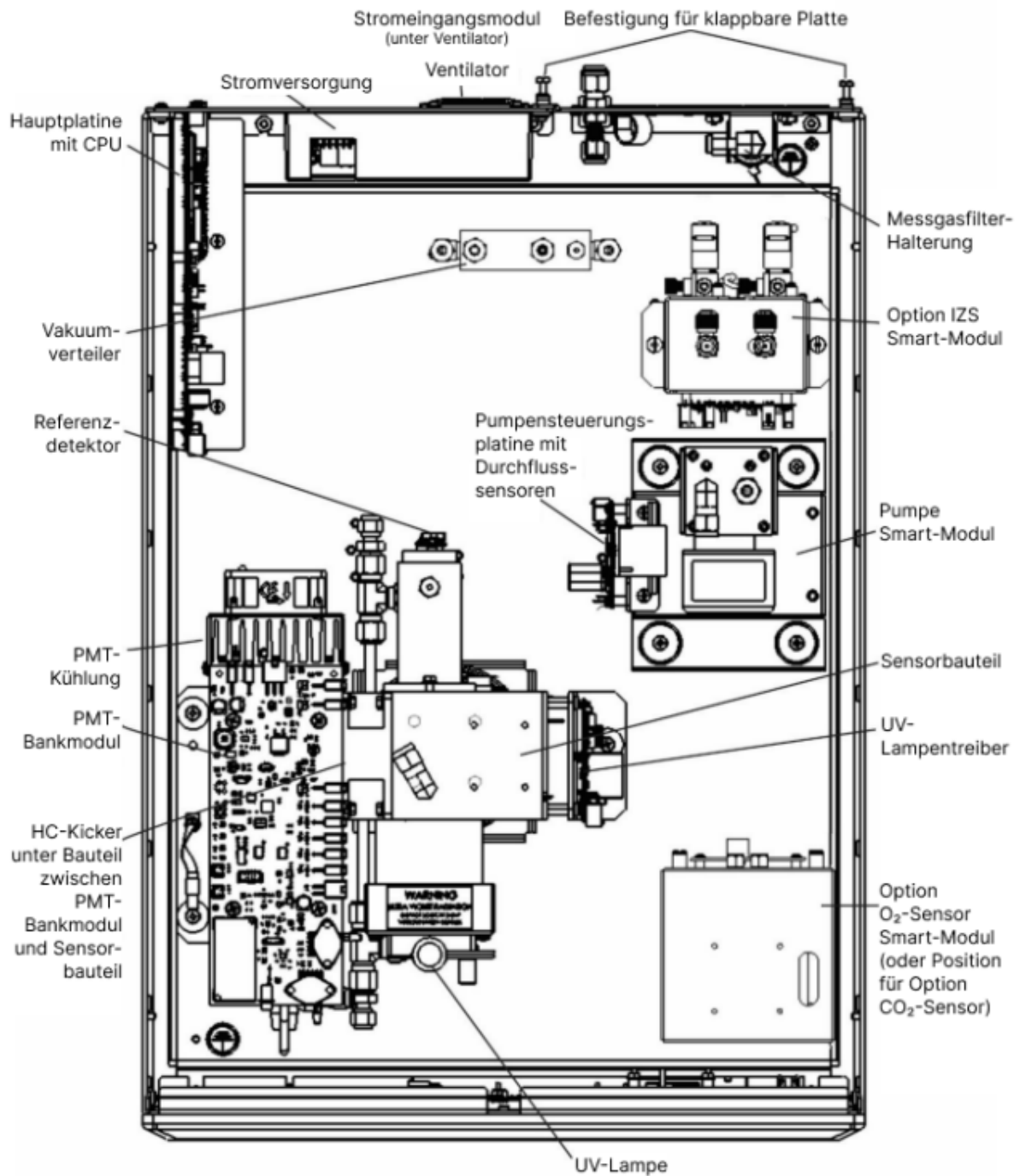
Abbildung 4: Aufbau des N100 Analysators
