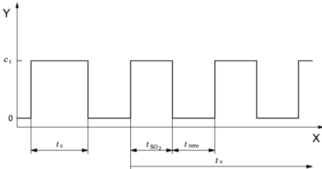
Abbildung 14: Prüfung des Mittelungseinflusses ( t_{SO_2} = t_{zero} = 45 \text{ s.} )
