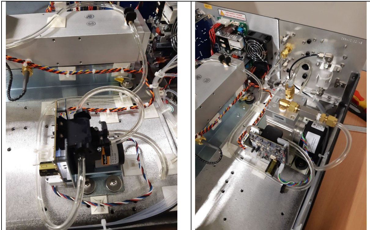
Abbildung 6: Geregelte Pumpe (links) und nicht geregelte Pumpe (rechts)
