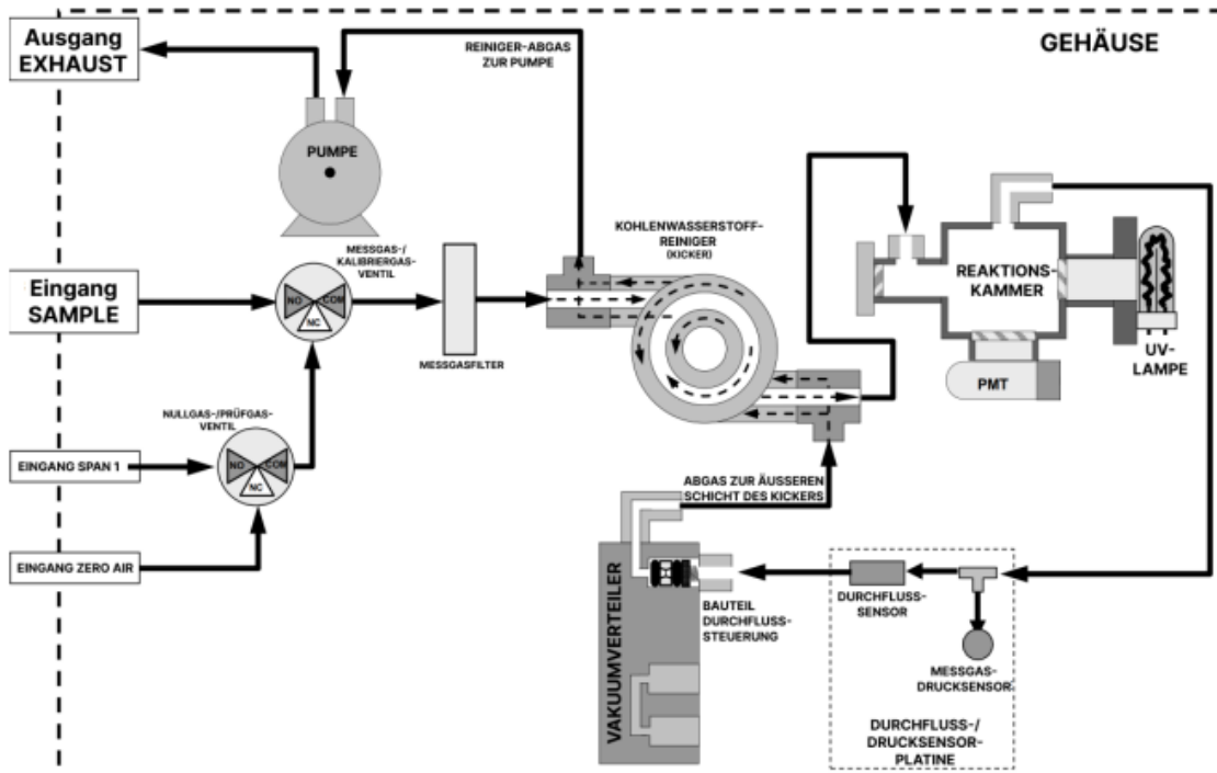
Abbildung 3: Pneumatisches Diagramm N100
