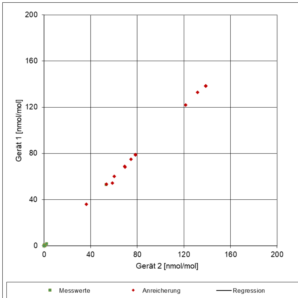
Abbildung 15: Grafische Darstellung der Vergleichsstandardabweichung im Feld
