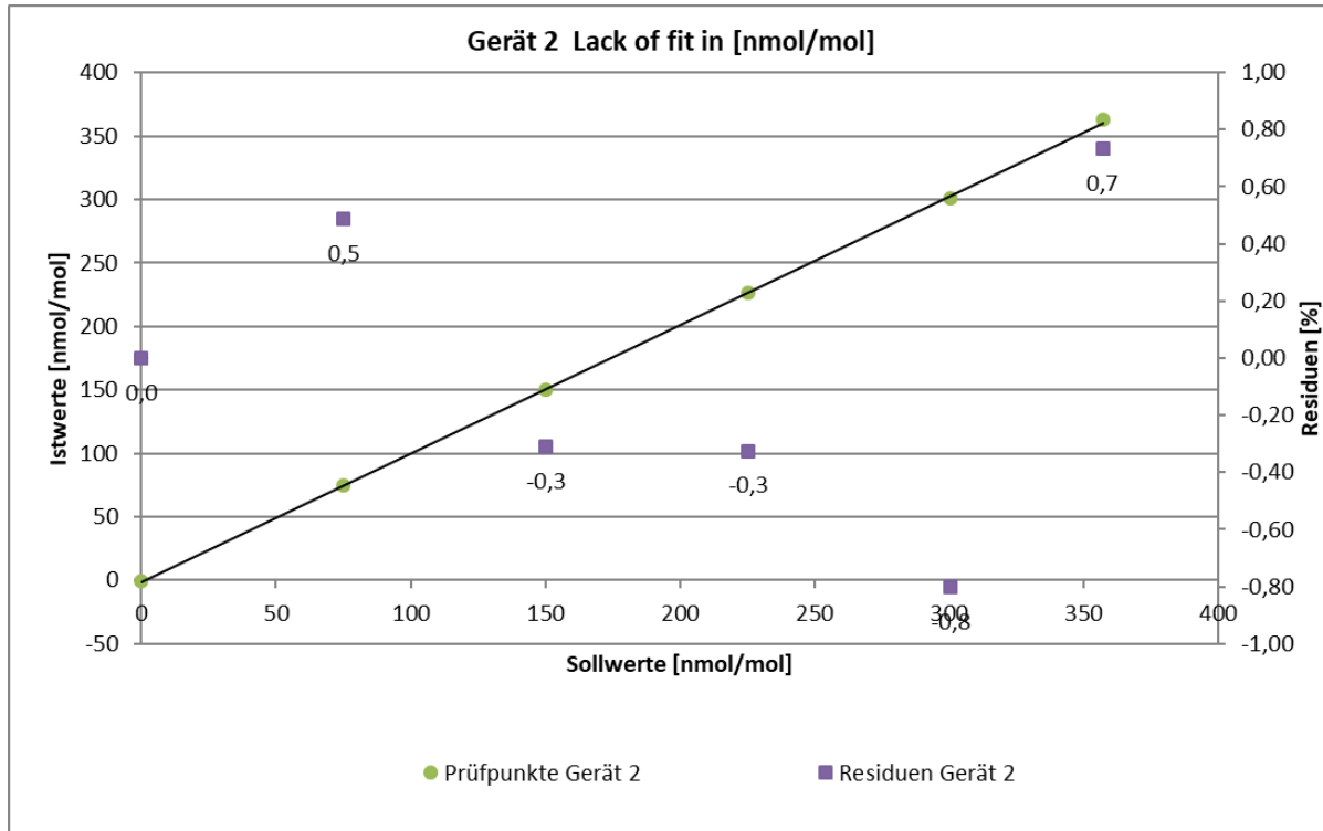
Abbildung 13: Analysenfunktion aus den Gruppenmittelwerten für Gerät 2
