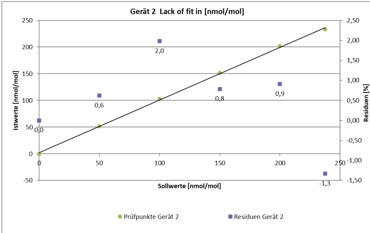
Abbildung 12: Analysenfunktion aus den Gruppenmittelwerten für Gerät 2
