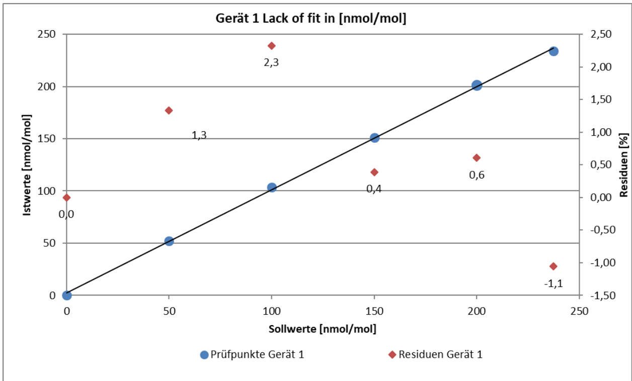
Abbildung 11: Analysenfunktion aus den Gruppenmittelwerten für Gerät 1
