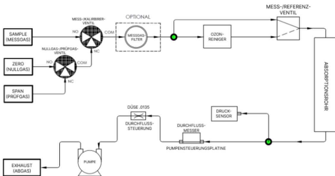
Abbildung 3: Pneumatisches Diagramm N400
