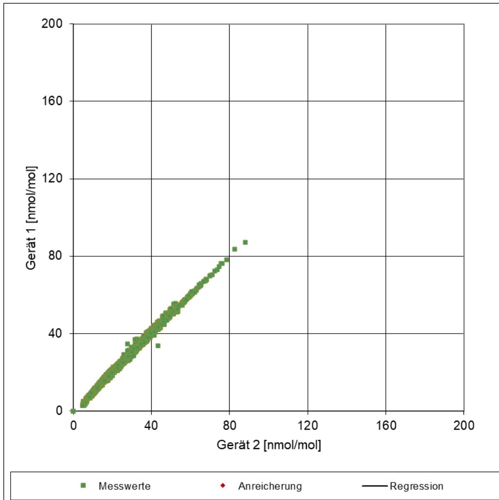
Abbildung 14: Grafische Darstellung der Vergleichsstandardabweichung im Feld
