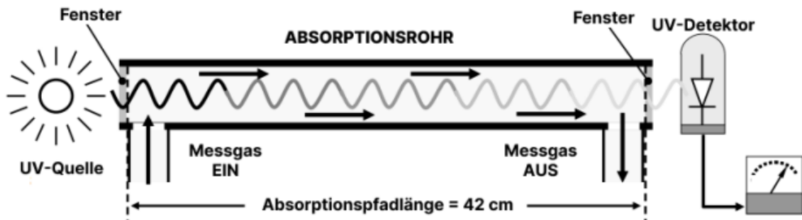
Abbildung 2: N400 Ozon Absorptionspfad
