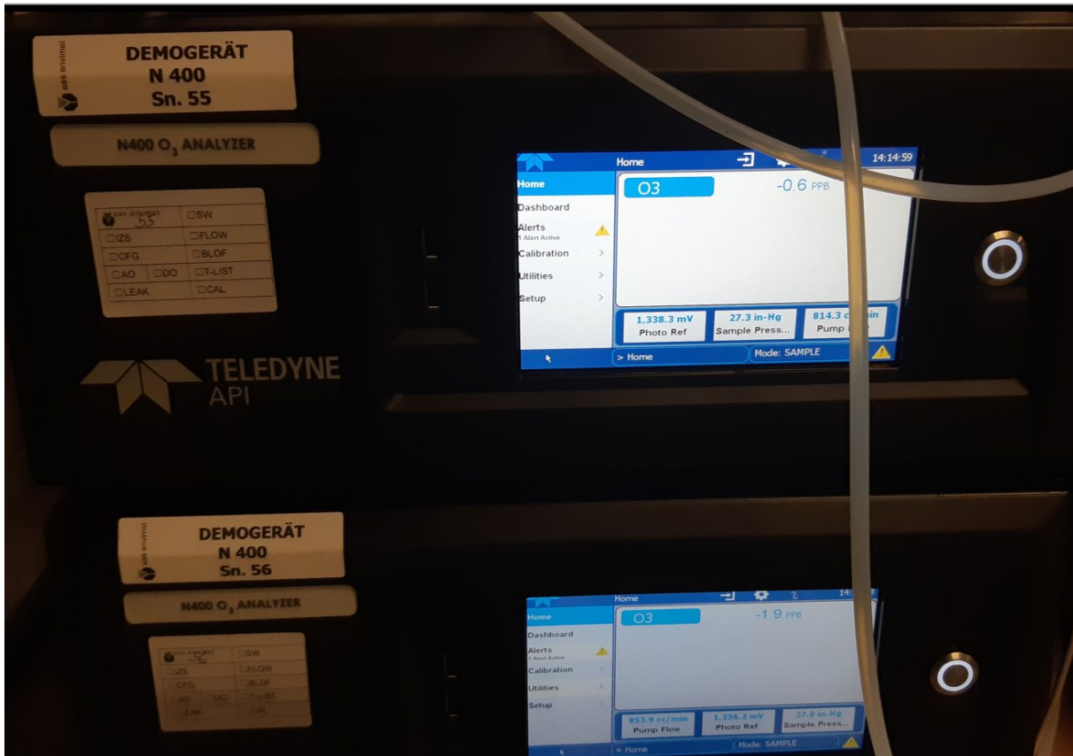
Abbildung 1: Darstellung des N400 Analysators
