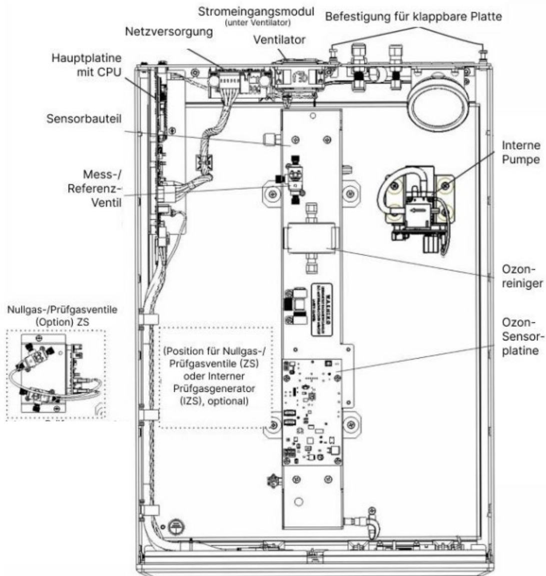
Abbildung 4: Aufbau des N400 Analysators
